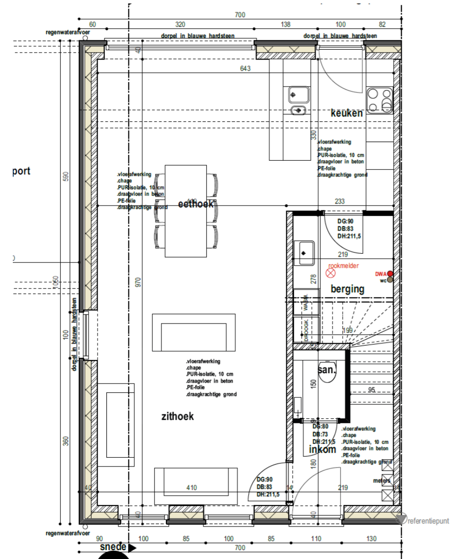
0 schaal 1:50
