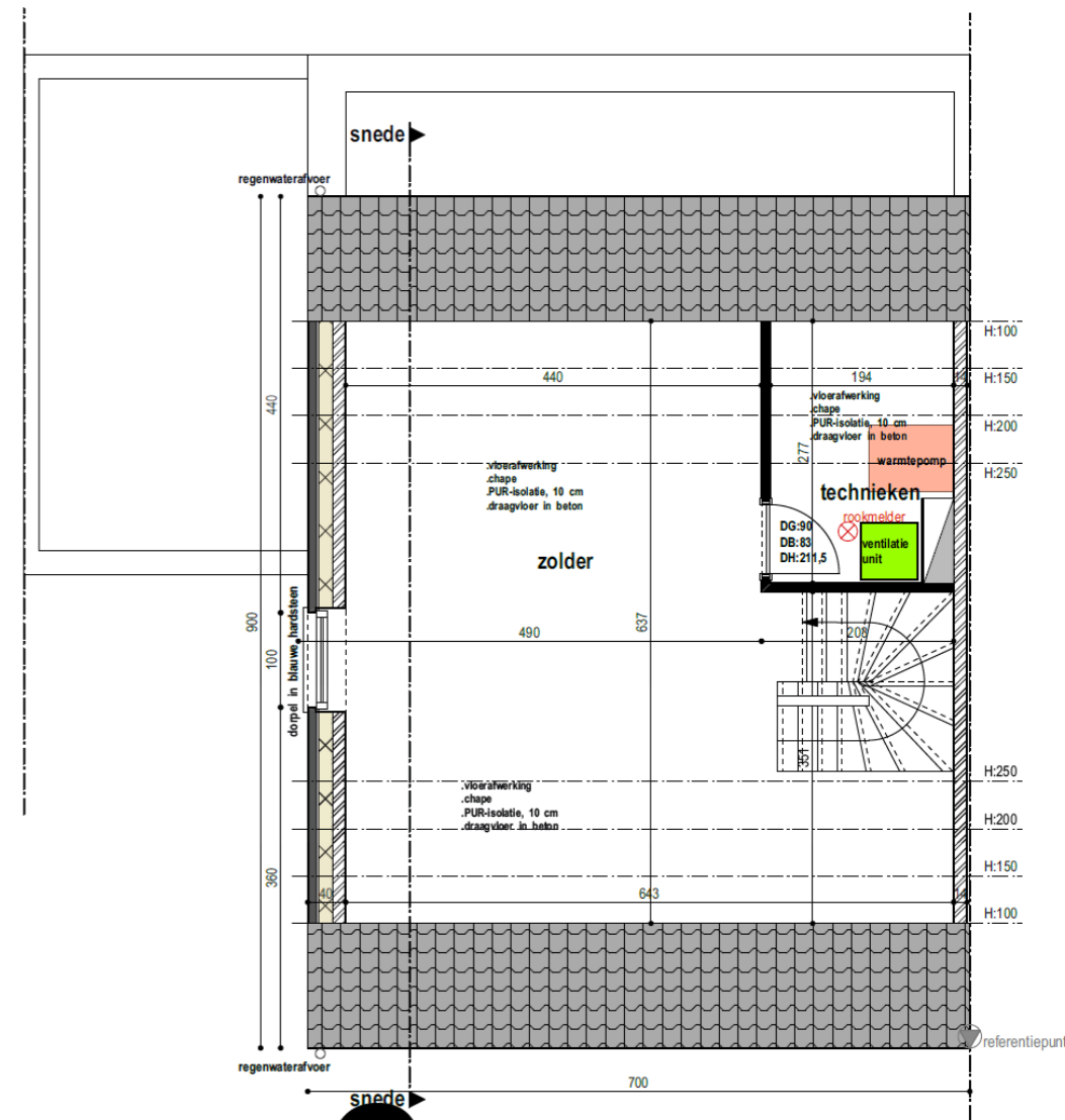
+2 schaal 1:50
